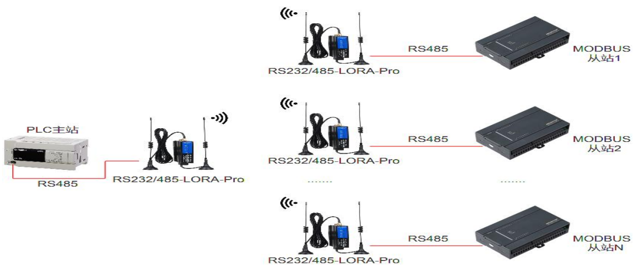
图 5.1.2.2 点对多通讯案例
