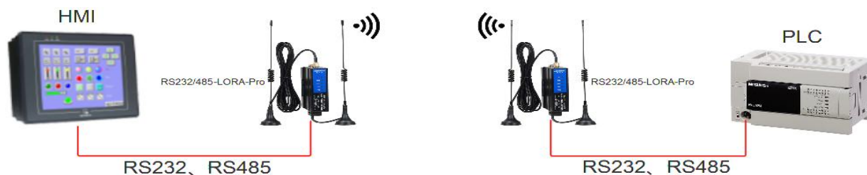
图 5.1.1.2 点对点单设备通讯
