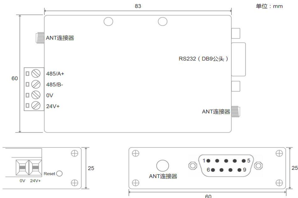
图 3.1 RS232/485-LORA-Pro 尺寸图
