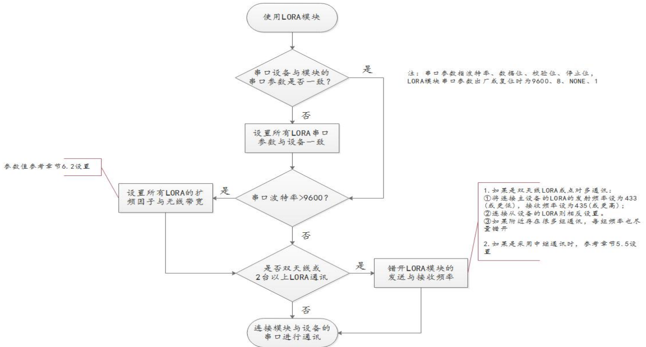
图 4.1 LORA 模块一般使用流程
