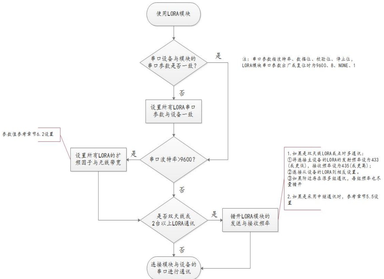
图 4.1 LORA 模块一般使用流程
