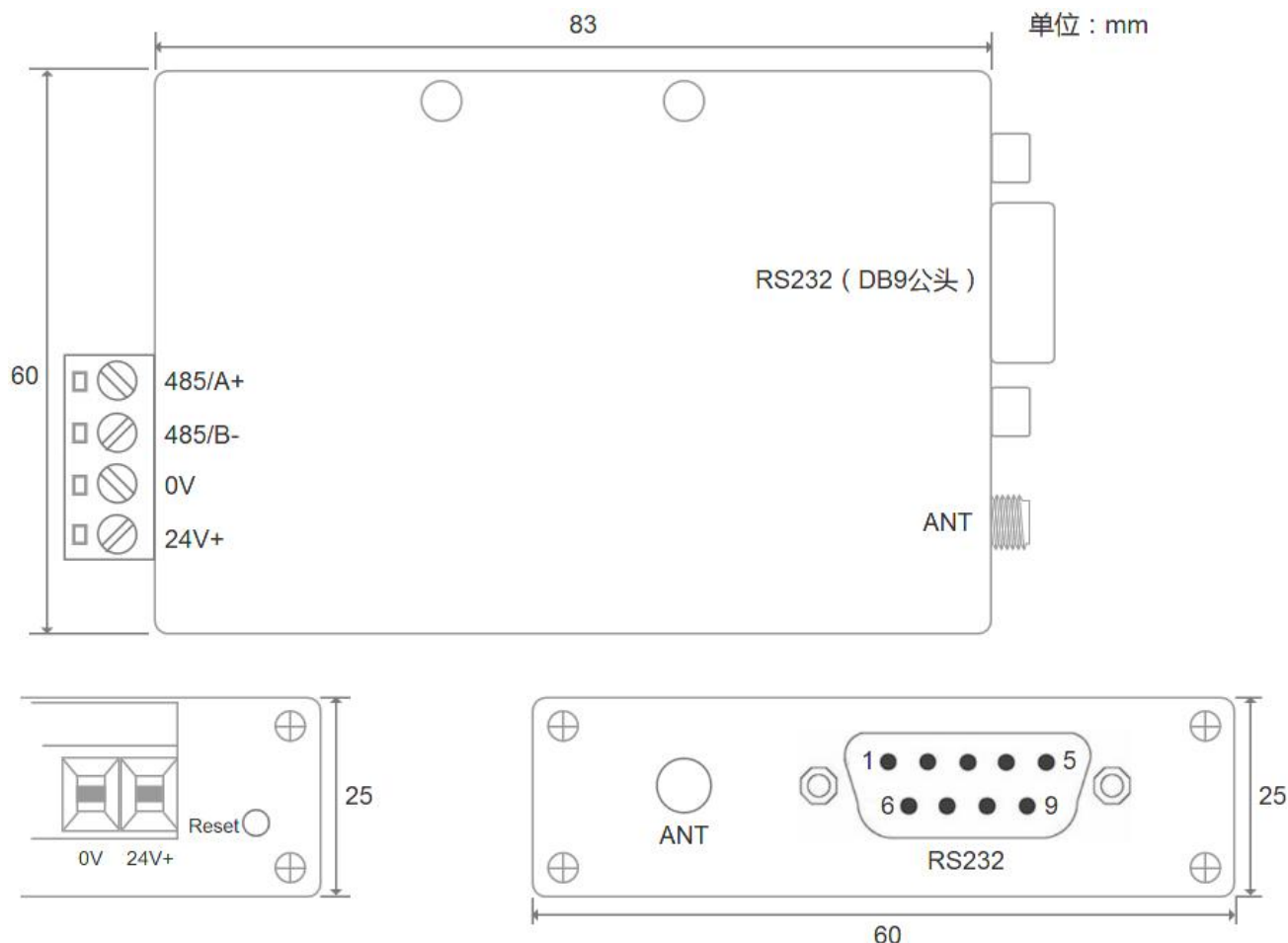
图 3.1 RS232/485-LORA-T 尺寸图
