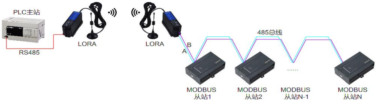
图 5. 1. 1. 3 点对点多设备通讯
