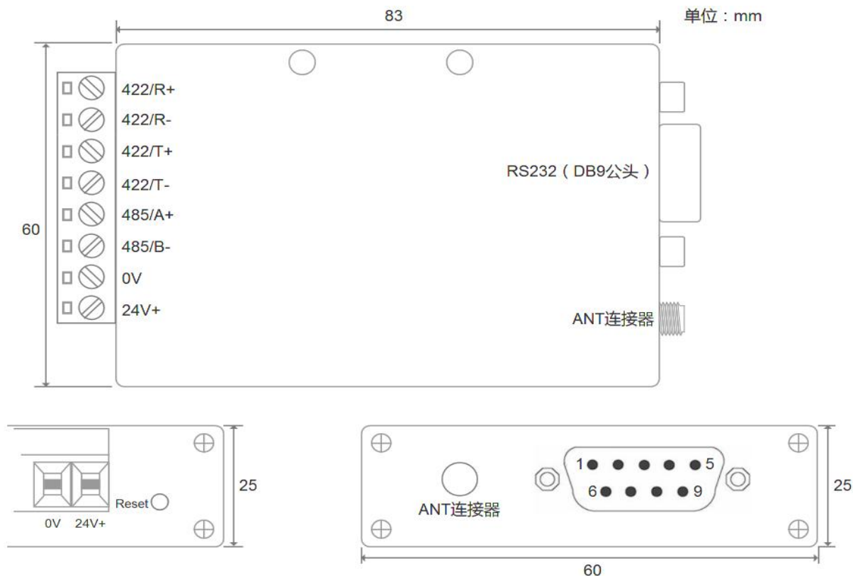
图 3.1 RS232/485/422-LORA 尺寸图
