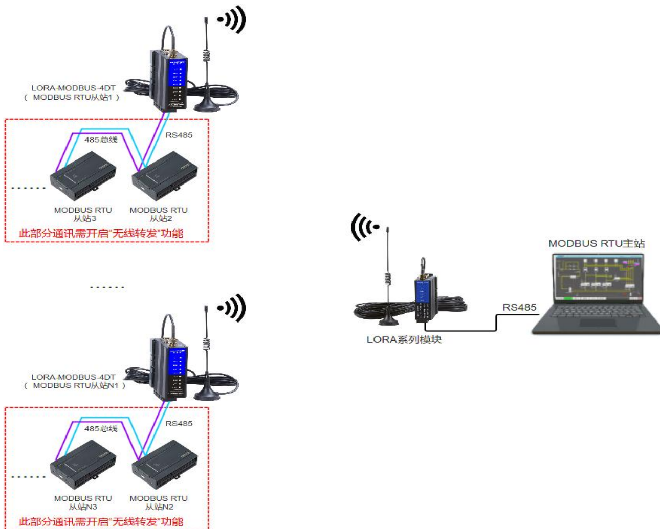
图 5.2.2 点对多点通讯
