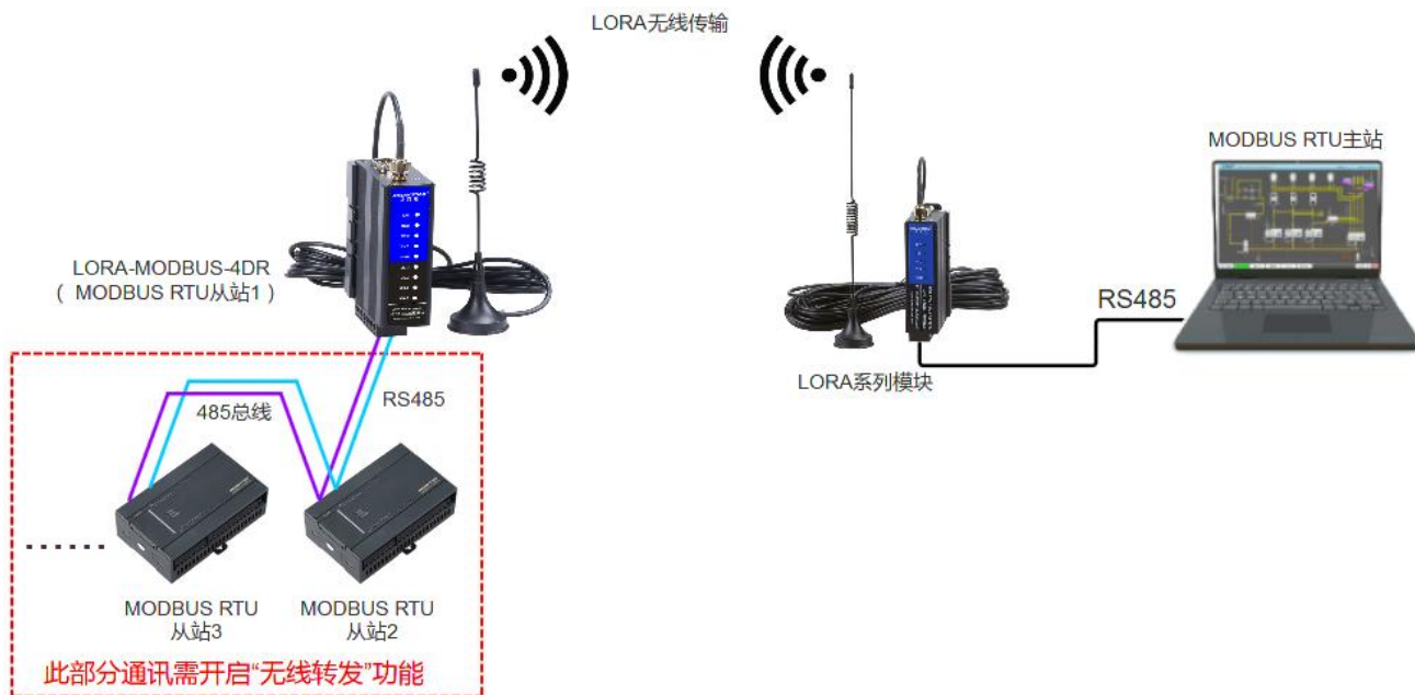
图 5.2.1 点对点通讯
