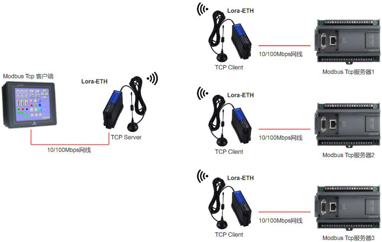
图 5.1.2.2 点对多通讯案例
