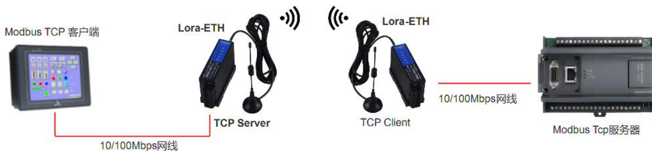
图 5.1.1.2 点对点单设备通讯
