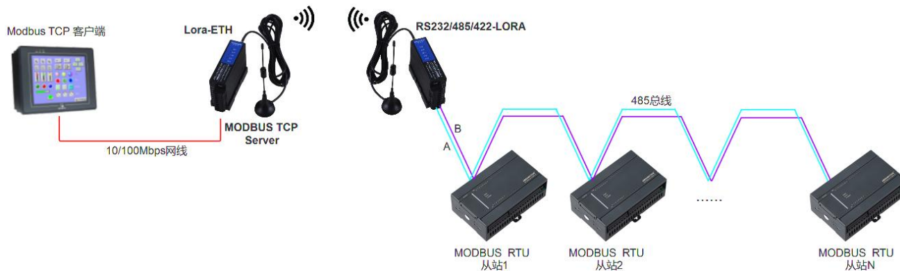
图 5.1.1.3 点对点多设备通讯
