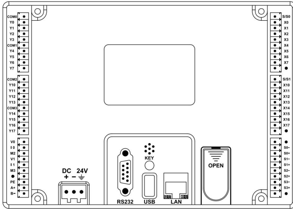
HM7R-32M 端子图
