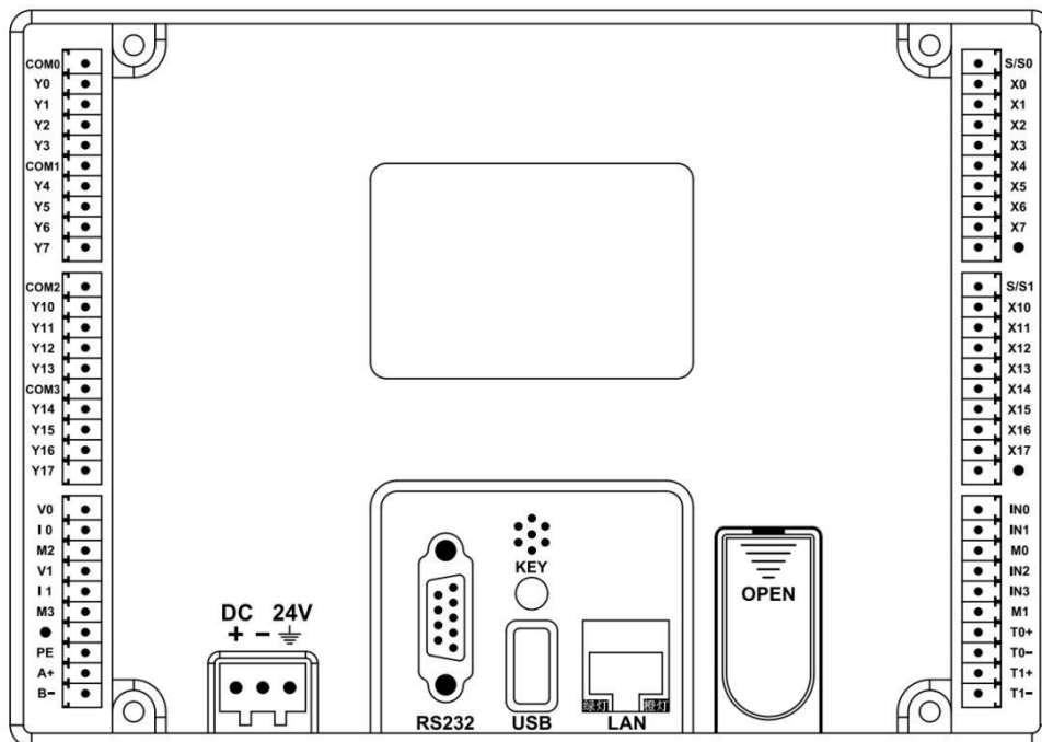
HM7N-32M 端子图
