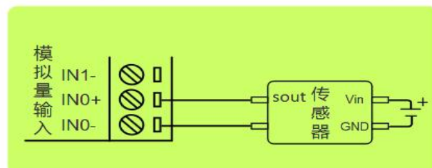
四线制传感器接法
