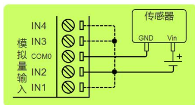
两线制传感器接法
