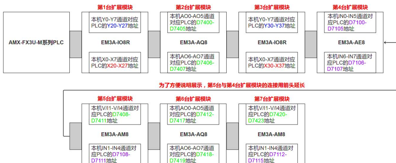
图 2.2 EM3A 扩展模块地址映射案例
