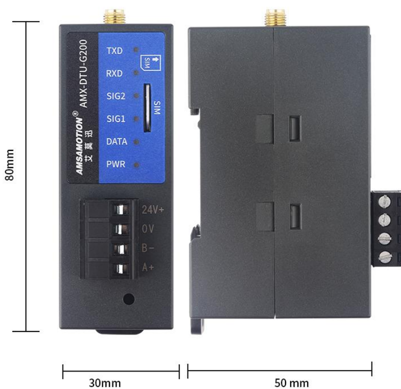
图 3.1 AMX-IOT-G200 模块尺寸图
