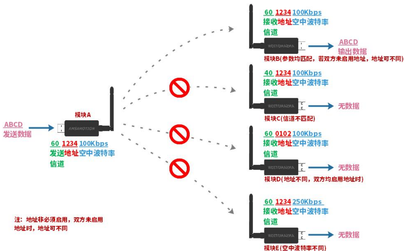
图 5.1.1 点对点发射
