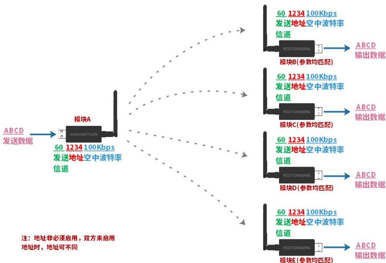
图 5.1.2 点对多发射
