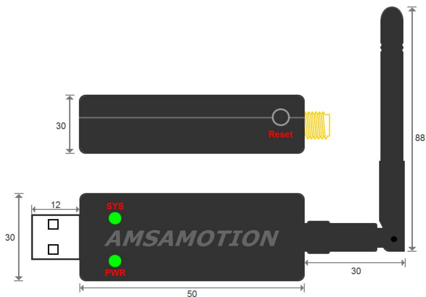
图 3.1 USB-RF24S 尺寸图
