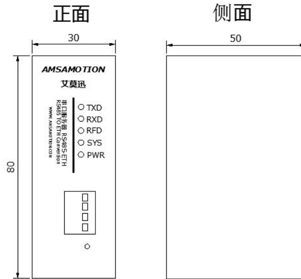
图 2.2 RS485-ETH 尺寸图
