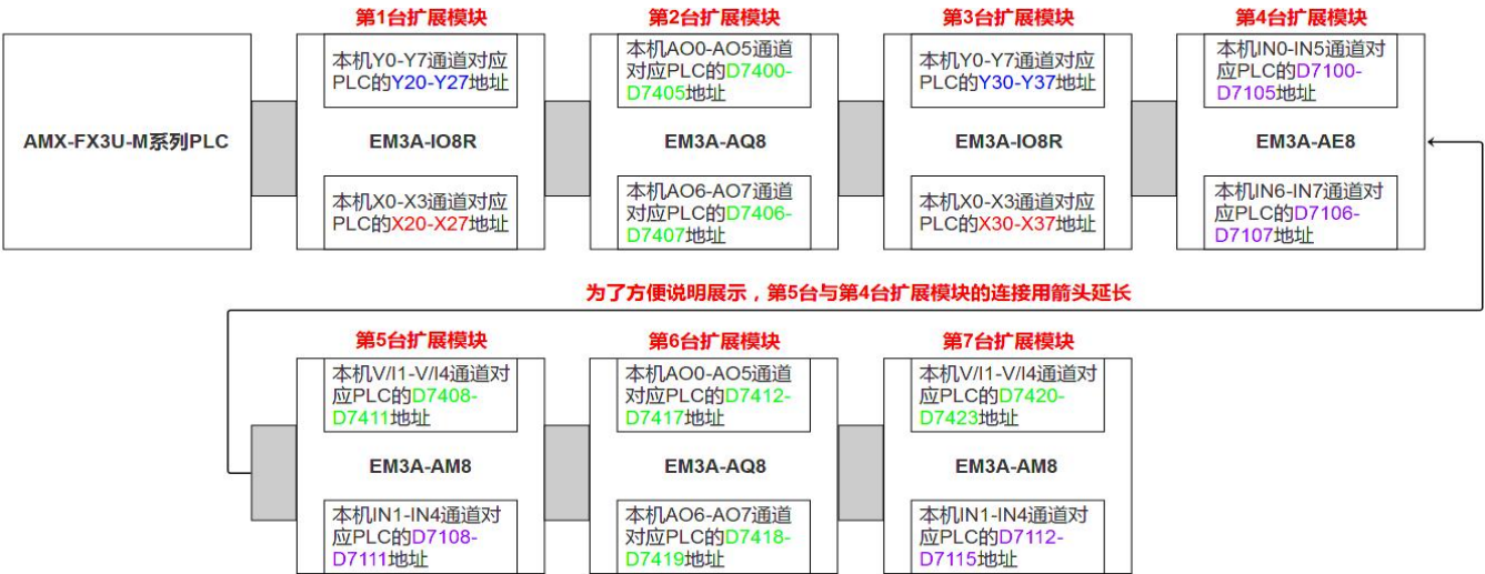
图 8.3.1 EM3A 扩展模块地址映射案例
