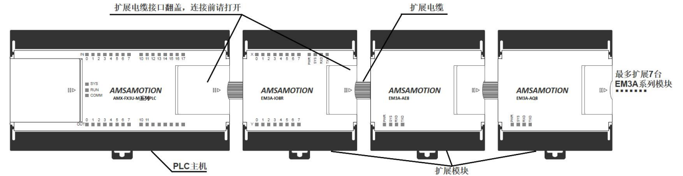
图 8.2 PLC 与扩展模块连接示意图
