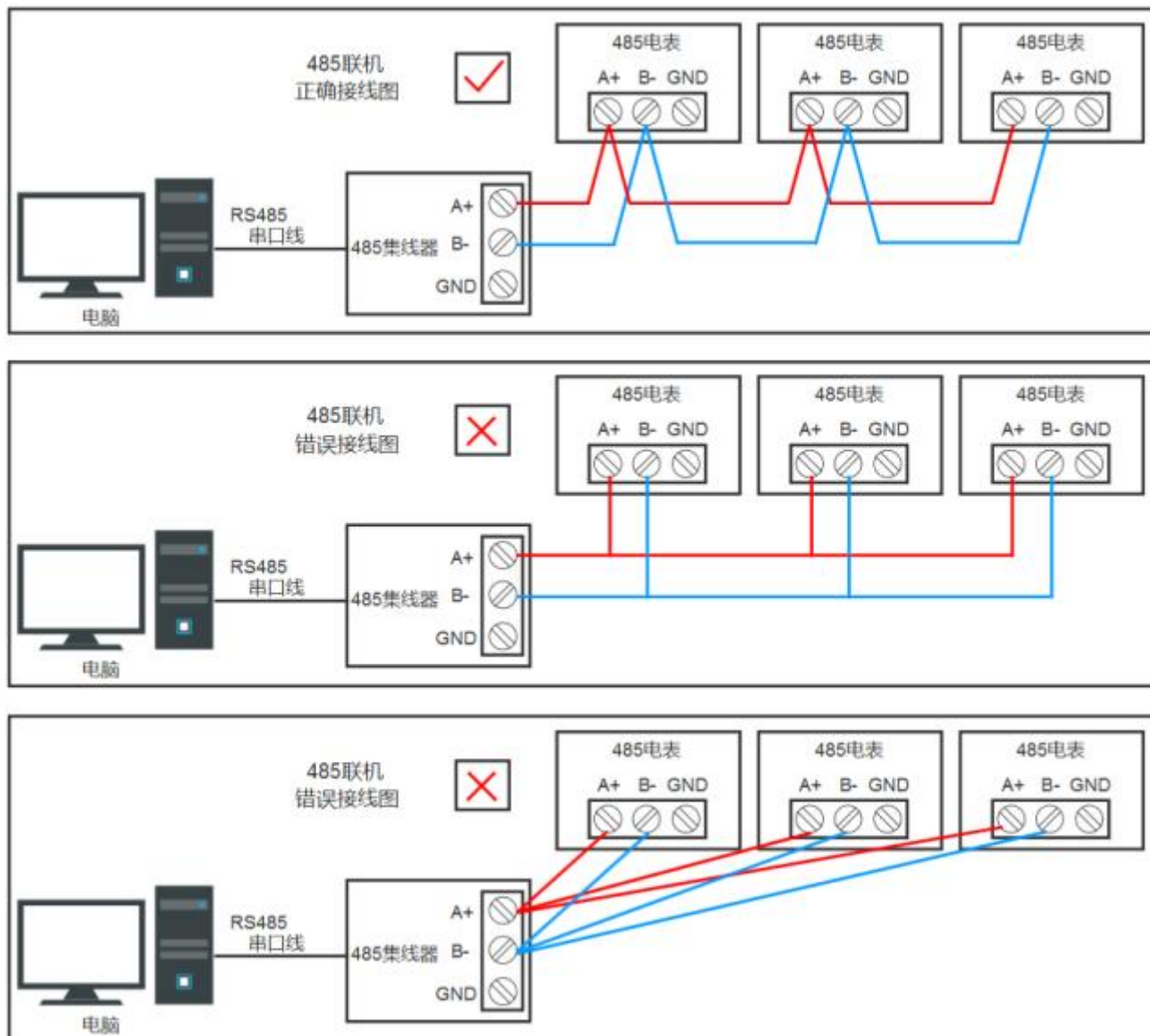
图 4.1 1P-485-4P+集线器总线接线说明
